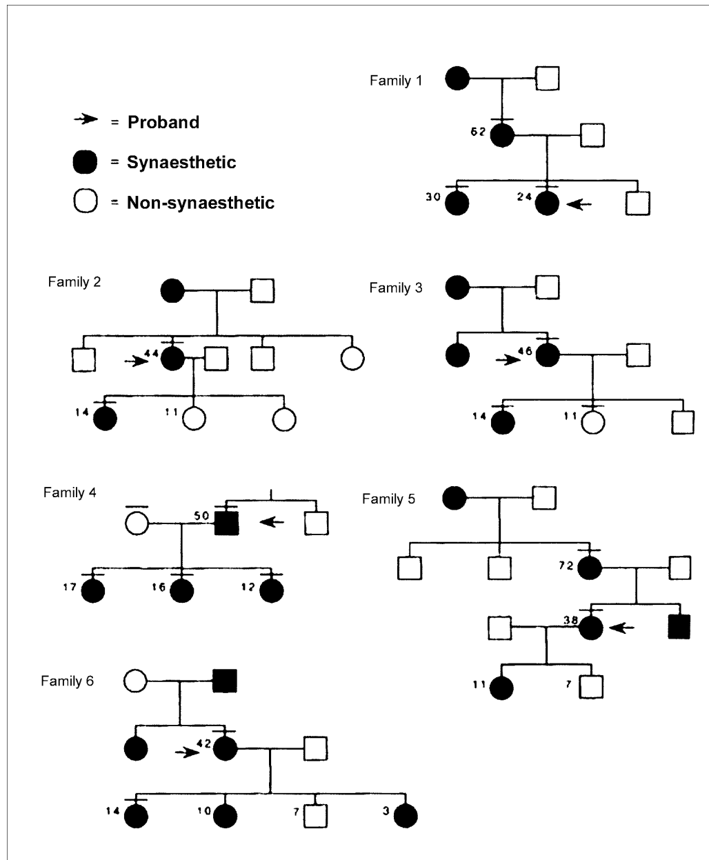
Kuva 2. Synestesian periytyvyystaulukko.
